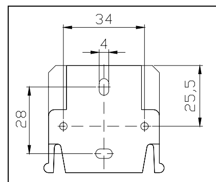
Рис.9 Шаблон для сверления
